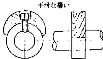
セットボルトの覆い
